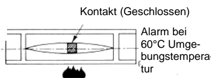
Abb.2: Langsame Erwärmung
